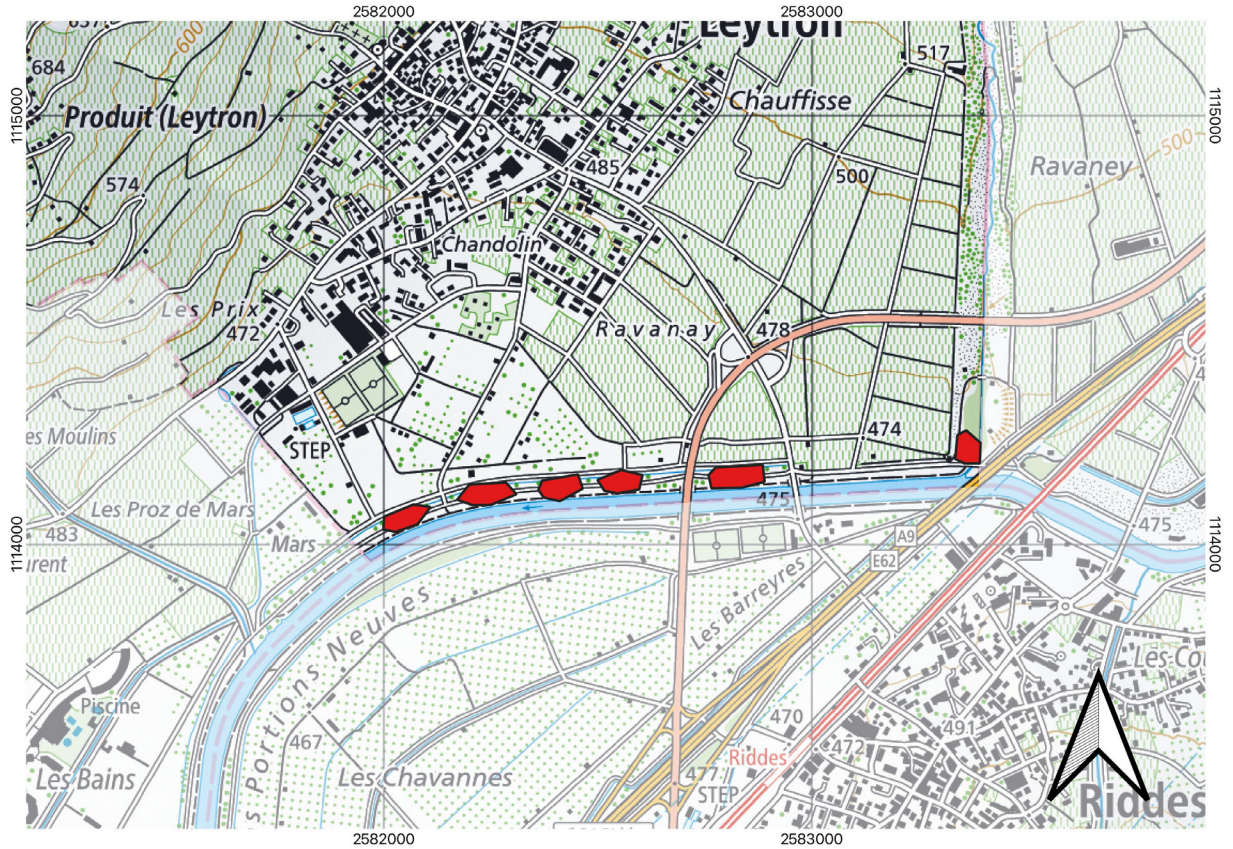
Fig. 24. Localisation des territoires de rossignol (N = 6) le long des berges.
