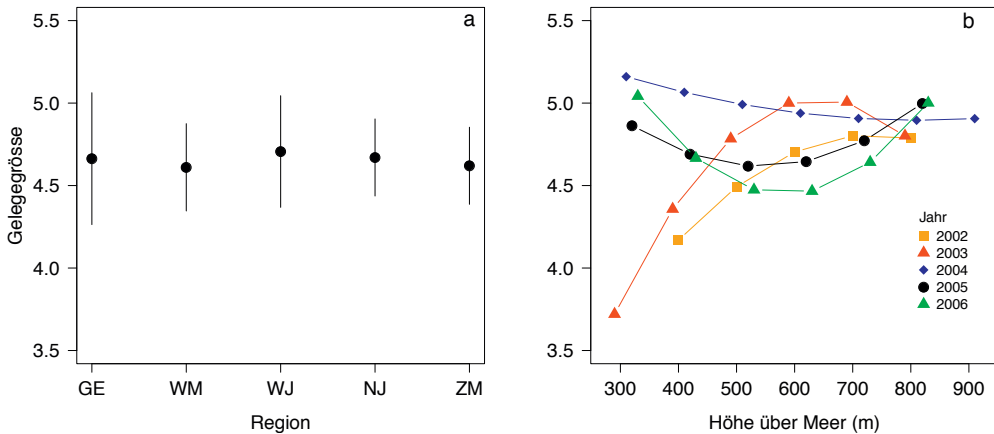
Abb. 6. Modellschätzwerte für (a) den Einfluss der Region (Genferseegebiet (GE), Westliches Mittelland (WM), Westlicher Jura (WJ), Nördlicher Jura (NJ) und Zentrales Mittelland (ZM)) auf die Gelegegröße ( \pm 95\% CI). Der Einfluss der Meereshöhe ist nicht in jedem Jahr derselbe. Die Schätzwerte sind berechnet für das Jahr 2005, die Region westliches Mittelland und das mittlere Legedatum (24. April). – Predicted mean clutch size ( \pm 95\% CI) in the different study areas (Lake Geneva Basin (GE), Western Plateau (WM), Western Jura Mountains (WJ), Northern Jura Mountains (NJ), Eastern Plateau (ZM)), (a) and in relation to altitude (b). The impact of altitude changed between years. The graph shows the predictions for the year 2005, the region Western Plateau and an egg-laying date of 24 April.
